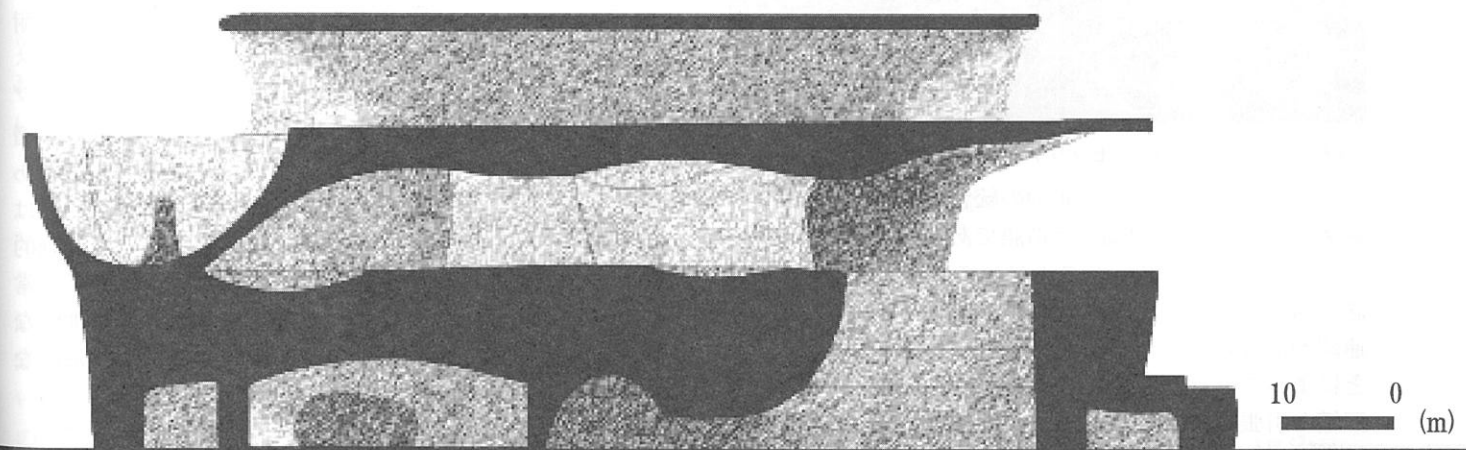
B-B' 断面
